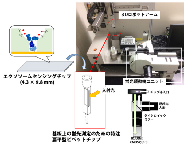
図2. エクソソーム自動分析計
