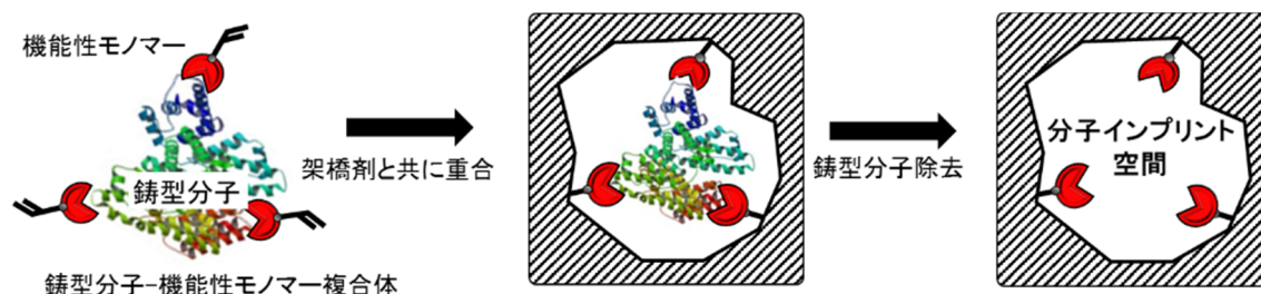
図 3. 分子インプリンティング技術の概念
